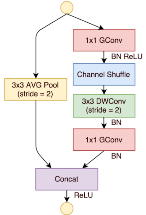
Figura 19. Unidad ShuffleNet [53]
