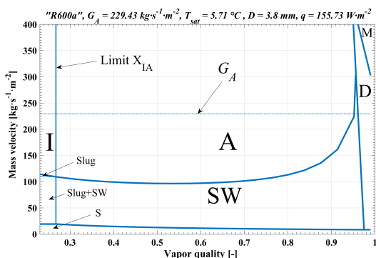
Figura 6. Mapa de patrones de flujo de la prueba D para el refrigerante R600a con una T_{sat} = 5,71\text{ °C} , D = 3,8\text{ mm} , q = 155,73\text{ W·m}^{-2} y G_A = 229,43\text{ kg·m}^{-2}·\text{s}^{-1}
