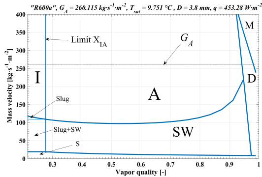
Figura 5. Mapa de patrones de flujo de la prueba C para el refrigerante R600a con una T_{sat} = 9,751\text{ °C} , D = 3,8\text{ mm} , q = 453,28\text{ W·m}^{-2} y G_A = 260,115\text{ kg·m}^{-2}·\text{s}^{-1}
