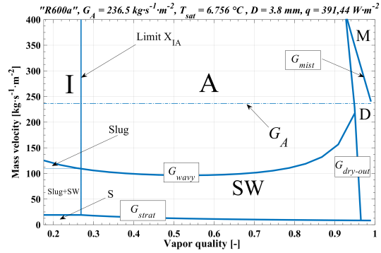
Figura 3. Mapa de patrones de flujo de la prueba A para el refrigerante R600a con una T_{sat} = 6,756 \text{ °C} , D = 3,8 \text{ mm} , q = 391,44 \text{ W} \cdot \text{m}^{-2} y G_A = 236,5 \text{ kg} \cdot \text{m}^{-2} \cdot \text{s}^{-1}
