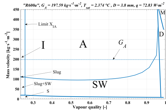
Figura 7. Mapa de patrones de flujo de la prueba E para el refrigerante R600a con una T_{sat} = 2,374\text{ °C} , D = 3,8\text{ mm} , q = 72,83\text{ W·m}^{-2} y G_A = 197,59\text{ kg·m}^{-2}·\text{s}^{-1}
