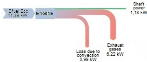
Figura 11. Sankey Diagram-Ecopais Gasoline
