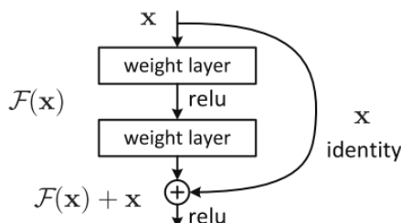
Figura 12. Bloque de la arquitectura ResNet [44]
