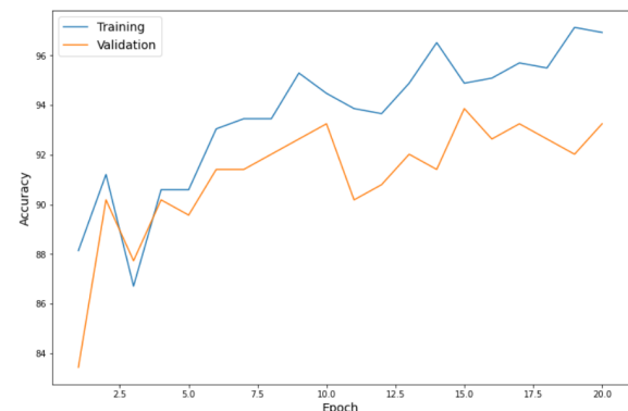
Figura 30. Accuracy: entrenamiento y validación del modelo
