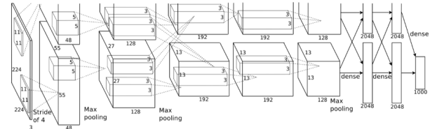
Figura 9. Arquitectura AlexNet [41]
