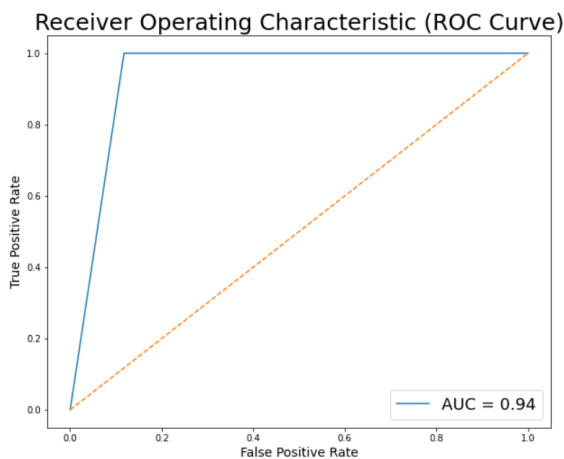
Figura 32. Curva ROC
