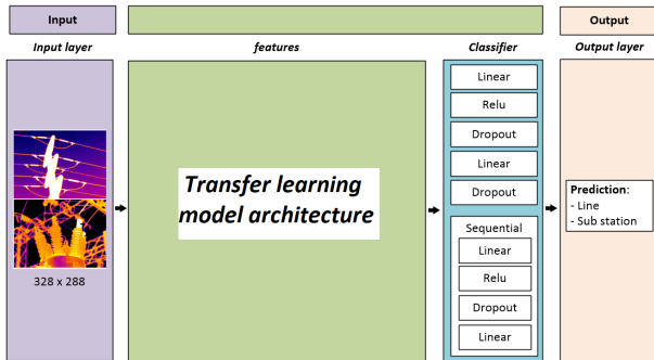
Figura 20. Arquitectura base
