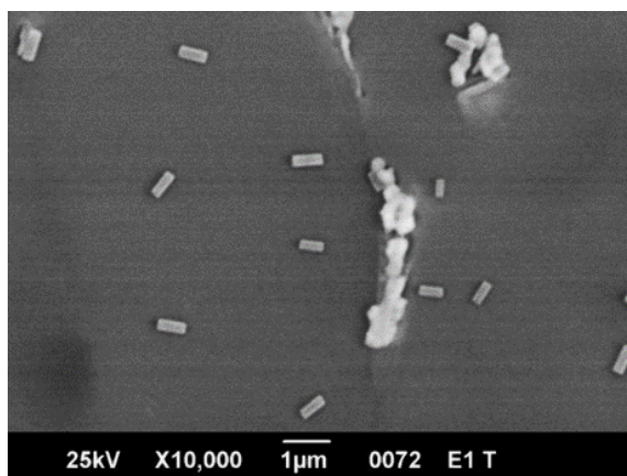
Figura 9. Micrografía SEM mostrando precipitados de \text{Al}_{6-7}\text{Mn} en muestras DC
